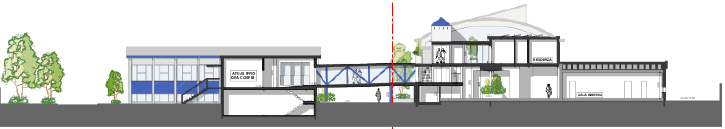
SEZIONE A-A
